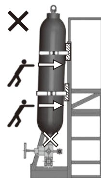
隙間に合わないスペーサーで 無理に固定すると給排油弁などに 無理な力がかかる
