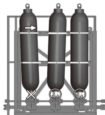
アクキュレータが傾いている クランプの中心がずれている クランプで締め込むことで給排油弁などに曲げモーメントが発生する
