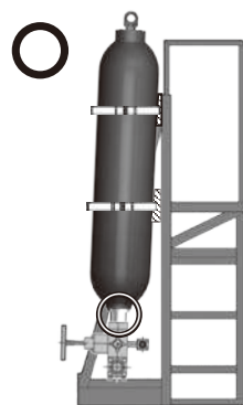
隙間にあったスペーサーを入れることで アクキュレータに無理な力がかからない
