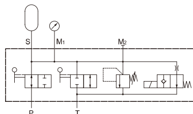
回路図
